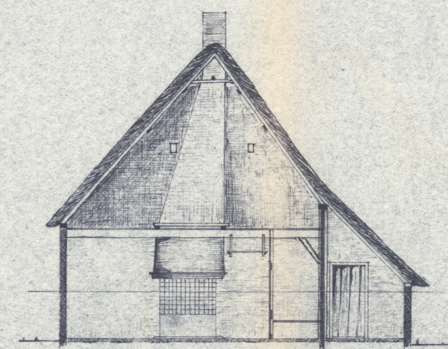
Doorsnede MM
