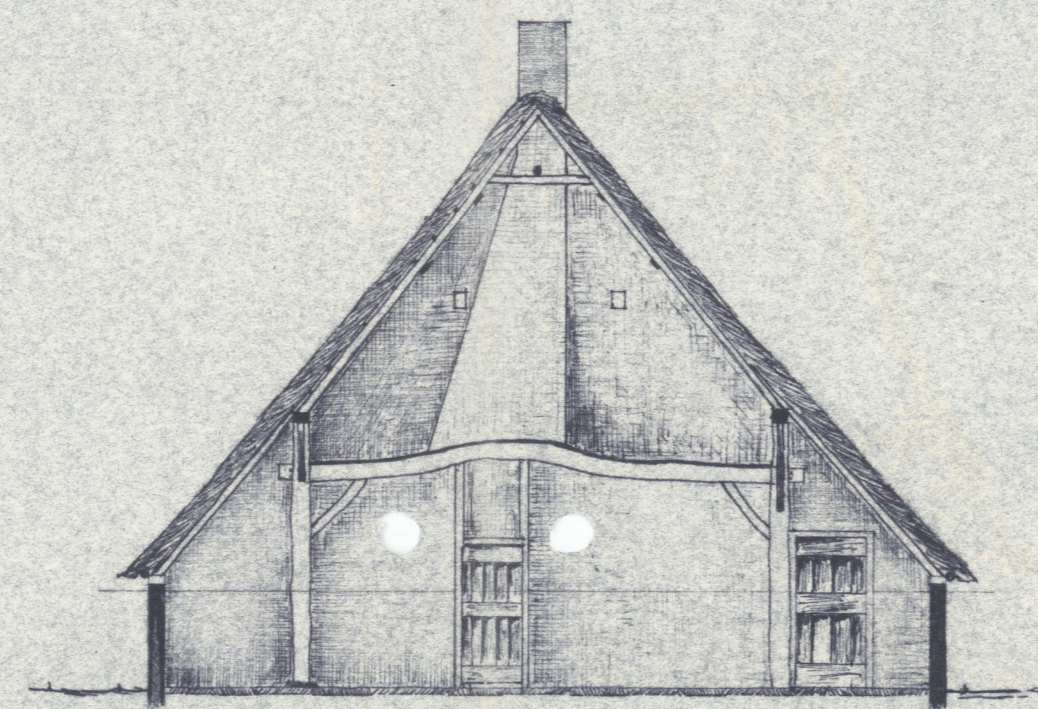
Doorsnede BB
