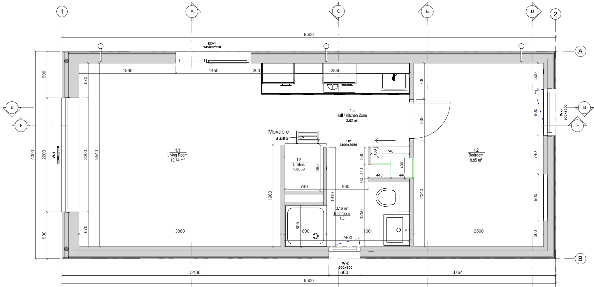
- Floor plan 1 : 30
